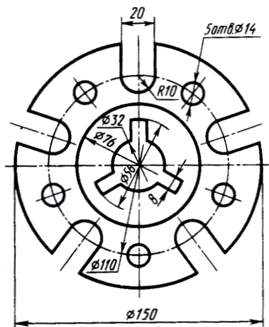
Фланец
