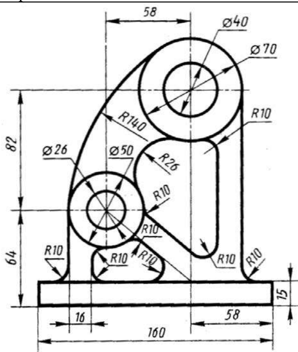
Станина
