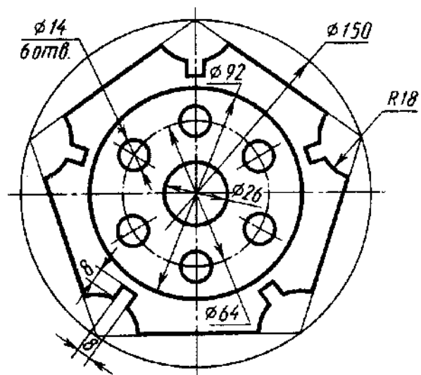
Крышка
