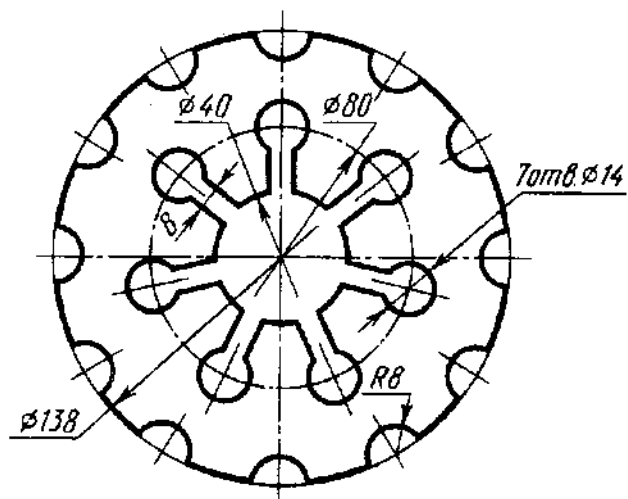
Прокладка
