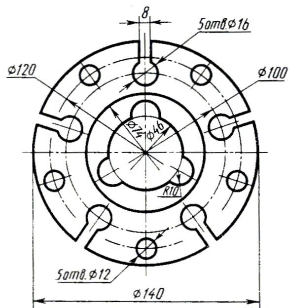
Прокладка
