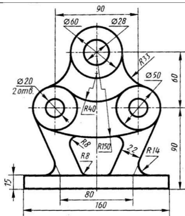
Станина
