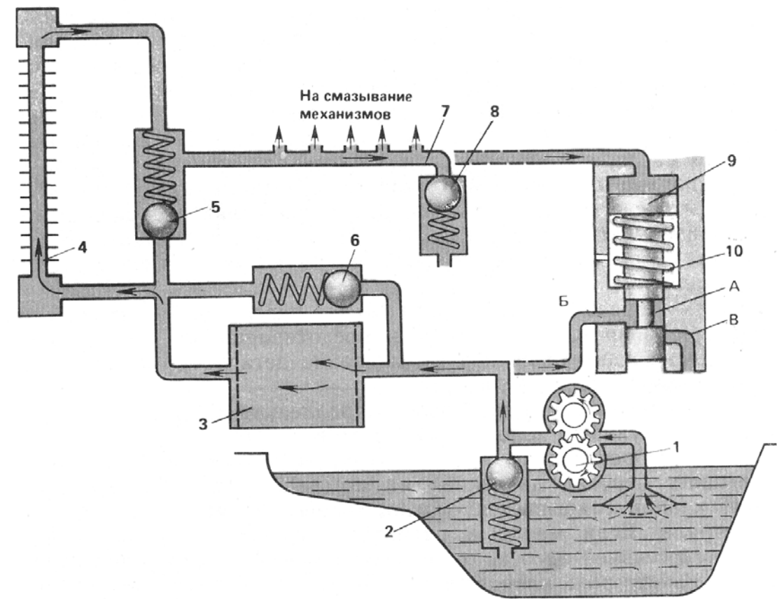
Р и с. 1. Принципиальная схема расположения клапанов системы смазки: 1 – масляный насос; 2 – редукционный клапан; 3 – маслоочиститель; 4 – радиатор; 5 – клапан термостат; 6 – перепускной клапан; 7 – магистраль; 8 – сливной клапан; 9 – дифференциальный клапан; 10 – пружина Таблица 4 – Отличительные особенности устройств, входящих в систему смазки двигателей
